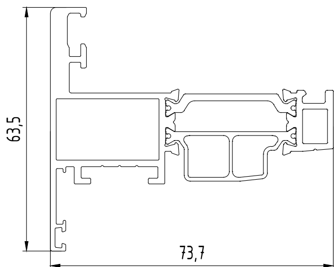
Профиль створки
