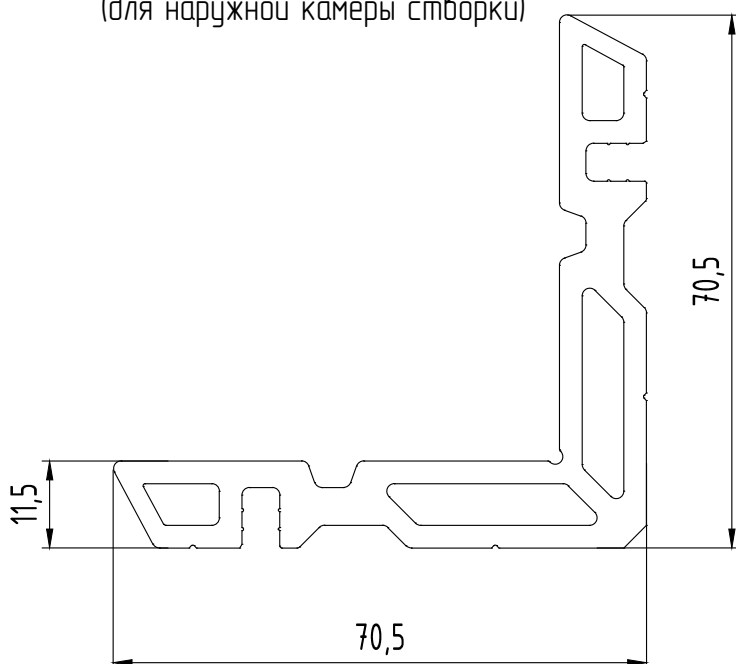
Закладная МП-45.08.02 l=6 мм (для наружной камеры створки)
